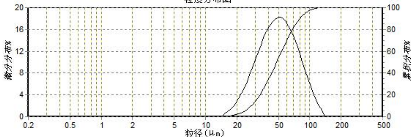
粒度分布图
